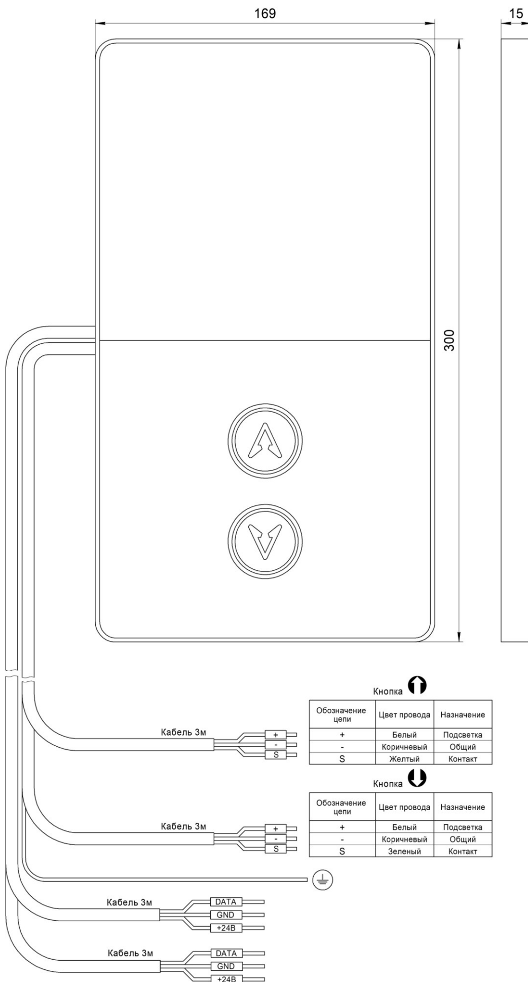
Рис.1 Внешний вид Вызывной пост ОНИКС НШЕК.468381.066
